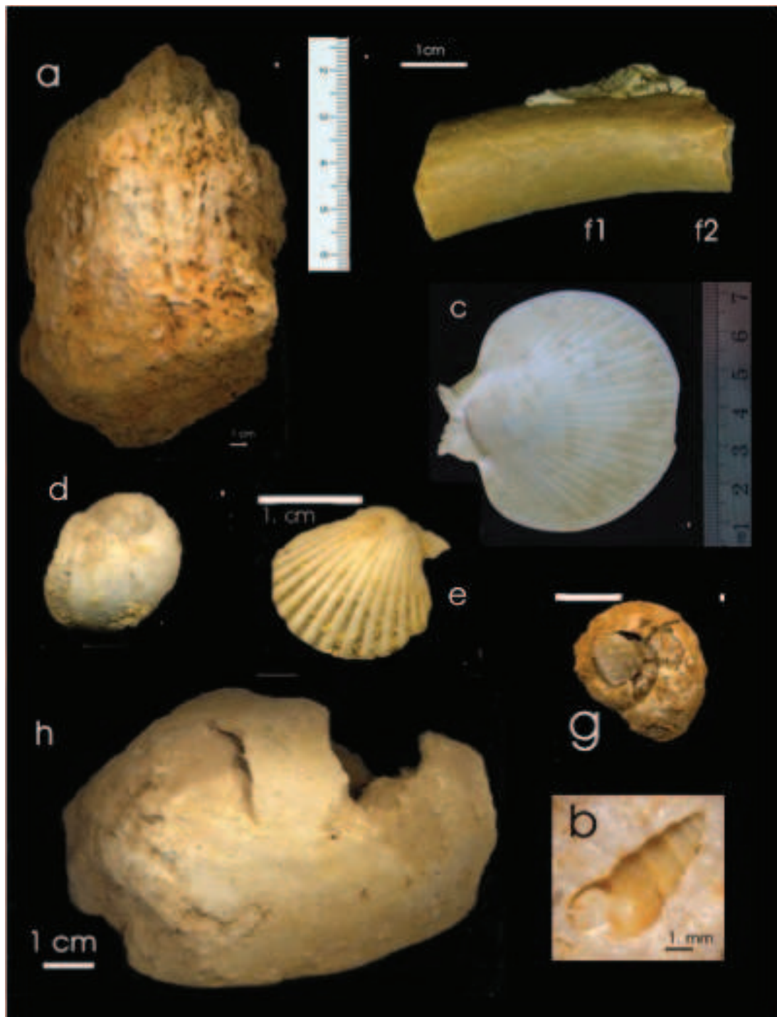
Fig. 4. Fòssils de la zona d'estudi: a) Fragment de trottoir de vermèts (Miocè. Puig de Son Seguí), b) Hydrobia sp. (Miocè. Puig de Son Seguí), c) Amusium cristatum (Pliocè inf.), d) Natica sp. (Pliocè mitjà. Comellar des Rafal), e) Chlamys sp. (Pliocè mitjà. Comellar des Rafal), f) fragment de costella de sirènid (Pliocè mitjà – sup. Barranc de sa Talaia), g) Gasteròpode pulmonat (Quaternari - Cova des Negret), h) Panopea glycymeris (Pliocè sup. Can Xerla – es Puget).
