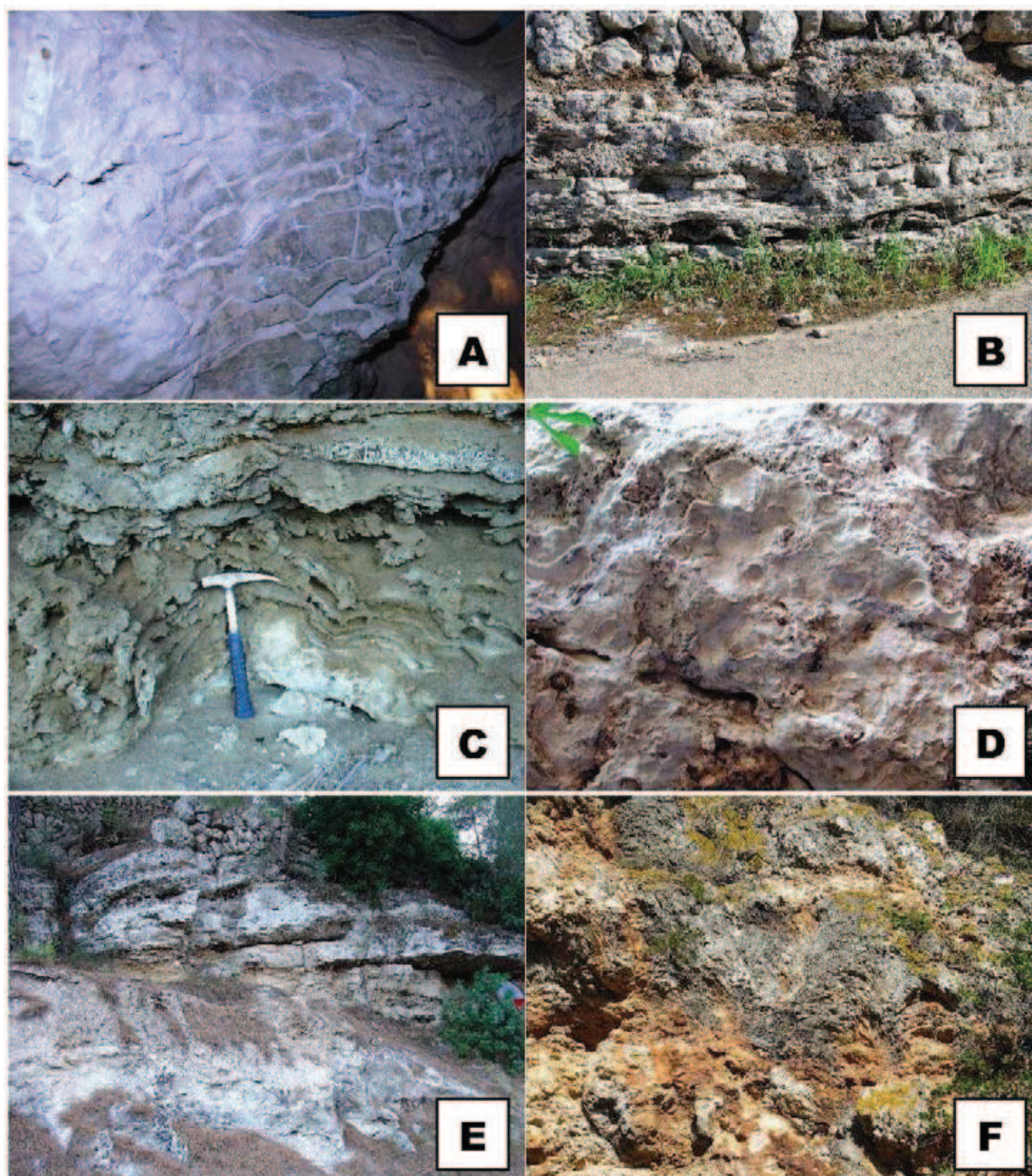
Fig. 3. Imatges de detall de les morfologies estromatolítiques del Complex Carbonàtic Terminal (Miocè) a la zona estudiada: A) Esquerdes de dessecació subaèria sobre estromatòlit (cova ermita de la Pau – Puig de Son Seguí); B) Laminació estromatolítica i grups trombolítics (Sencelles); C) Doms amb forta recristal·lització tipus fàcies Pont d’Inca (Cas General); D) Laminació amb doms centimètrics tipus LLH (Cas General); E) Conglomerats tasconats passant lateralment a calcàries amb estromatòlits (Son Sineu); F) Calcàries amb doms i ripples (Son Sineu).
