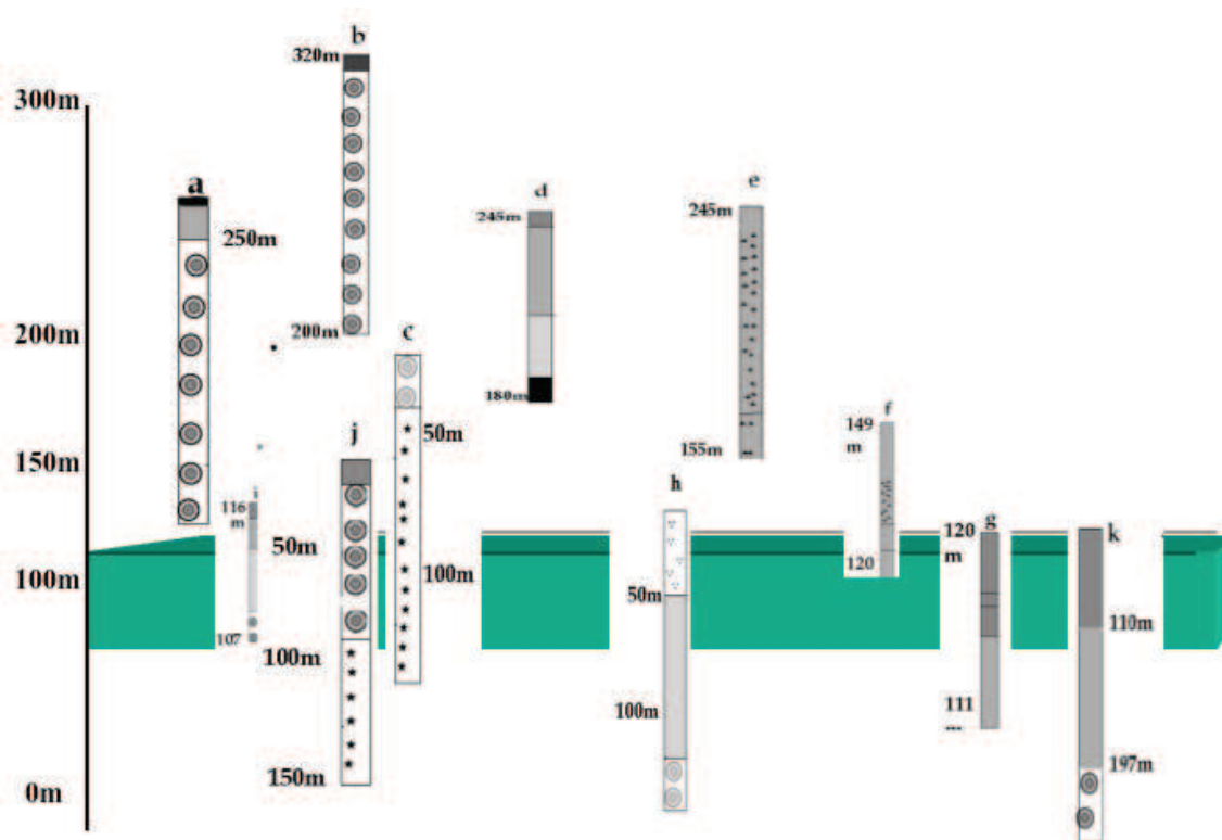
Fig. 7. Columnes estratigràfiques sintètiques corresponents a la zona estudiada i gràfica comparativa amb altres localitats de Mallorca: a) Puig de Son Seguí (Oest), b) Puig de Son Seguí (cim), c) Comellar des Abatzers (sondeig, Benedicto, 1994), d) Puig de Sta. Eugènia (Monument), e) sa Creueta, f) Es Puget, g) sa Cova Monja, h) es Pou Nou (sondeig. Benedicto, 1994), i) Pontiró - Cas General, j) sa Talaia (sondeig. Benedicto, 1994), k) Inca (sondeig. Colom, 1967).
