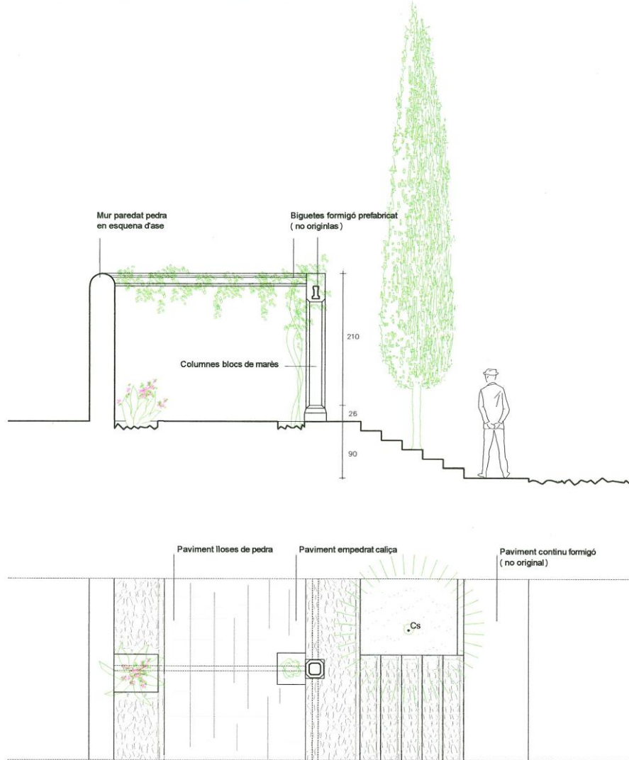
Figura 329. Pèrgola del jardí. Secció i planta. Elaboració: M. I. Riera Pinya.
