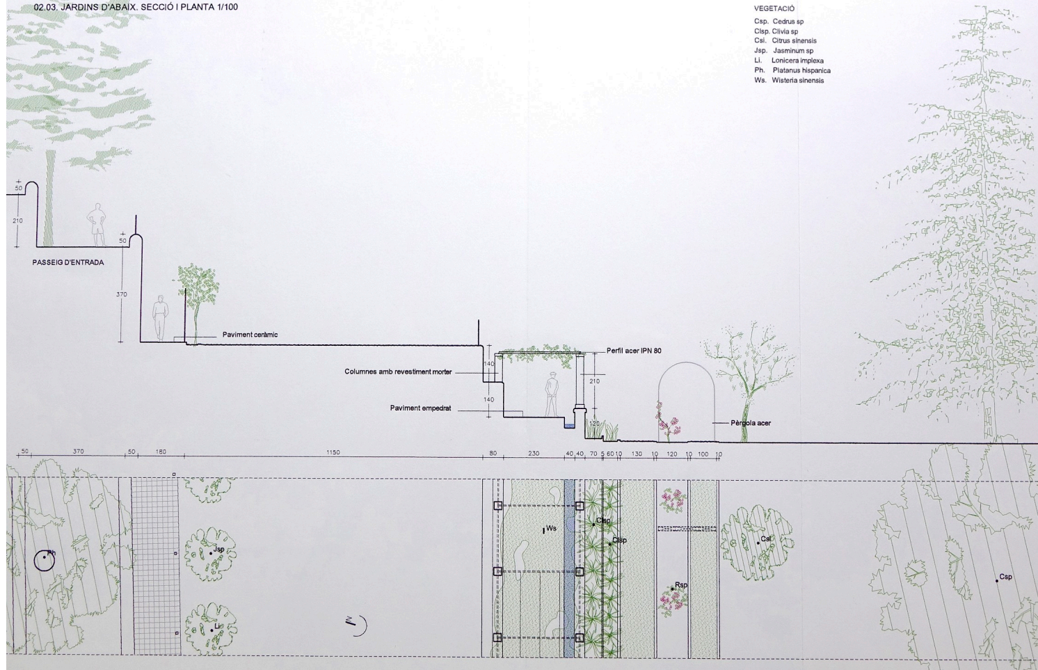
Figura 149. Secció i planta del jardí de baix. Elaboració: M. I. Riera Pinya.
