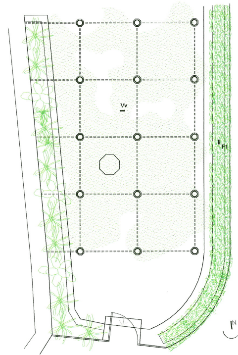
Figura 143. Pèrgola del jardí de dalt. Secció i planta. Elaboració: M. I. Riera Pinya.
