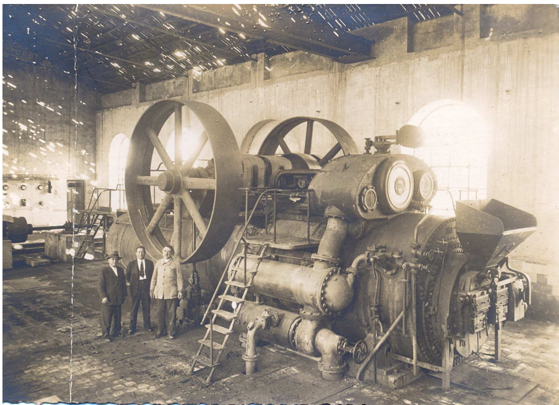
Motor de gas de l'empresa El Gas S.A. -1917- (Arxiu Municipal de Sóller)
