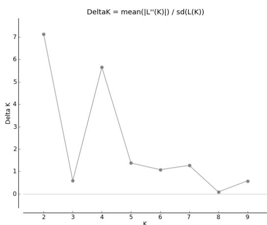
Figura 1. Variación del estadístico \Delta K , que infiere el número de clusters genéticos, asignando un valor probable de K=2 .
