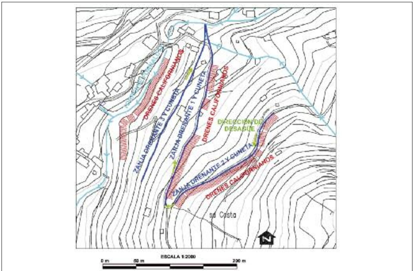
Figura 12. Medidas de estabilización de la ladera. El objetivo fundamental es favorecer el drenaje de la misma, para lo que se propone la ejecución de una serie de zanjas y cunetas drenantes, así como una batería de drenes californianos. El agua recogida se evacuaría hacia el torrente que discurre en el margen septentrional del deslizamiento que, a su vez, drena hacia el torrente de Fornalutx.
