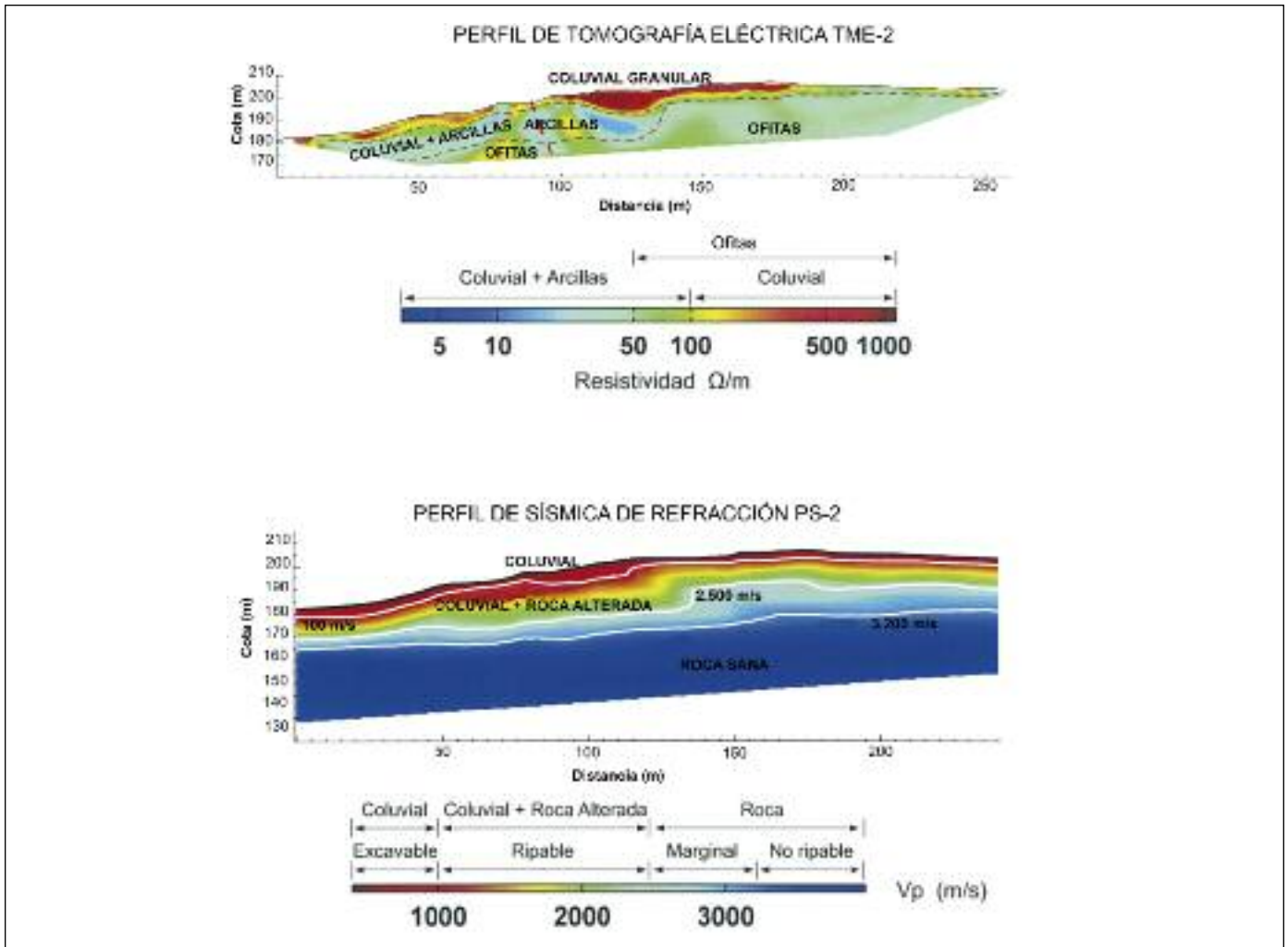
Figura 7. Perfiles de sísmica de refracción y tomografía eléctrica. En ambos perfiles se observa un nivel superficial, de unos 20 m de potencia, que corresponde a materiales granulares y arcillosos muy alterados, que se dispone sobre un sustrato rocoso inalterado. La superficie de deslizamiento podría corresponder con el contacto entre estos dos tipos de materiales, que parece seguir en profundidad la topografía de la ladera.
