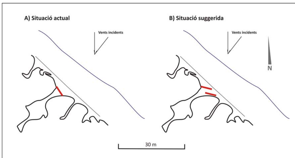
Figura 203: Representació esquemàtica de la disposició i orientació de les trampes suggerida envers a la component dels vents principals incidents.
