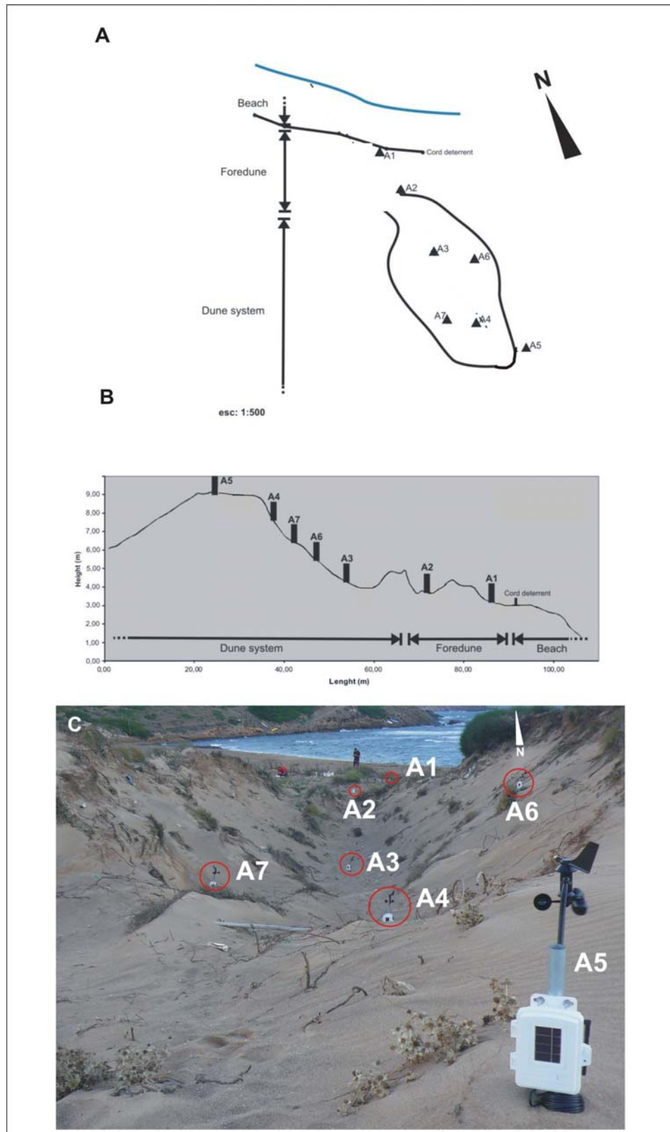
Figura 54: Disposició i localització dels anemòmetres desplecats en les campanyes realitzades al blowout de Cala Tirant (Menorca). A la figura A un esquema en planta de la localització de cada un dels sensors, al B la seva localització vista en perfil – sobre el perfil topogràfic – longitudinal del blowout , i al C una imatge presa in situ al camp, al llarg de l'experiment.
