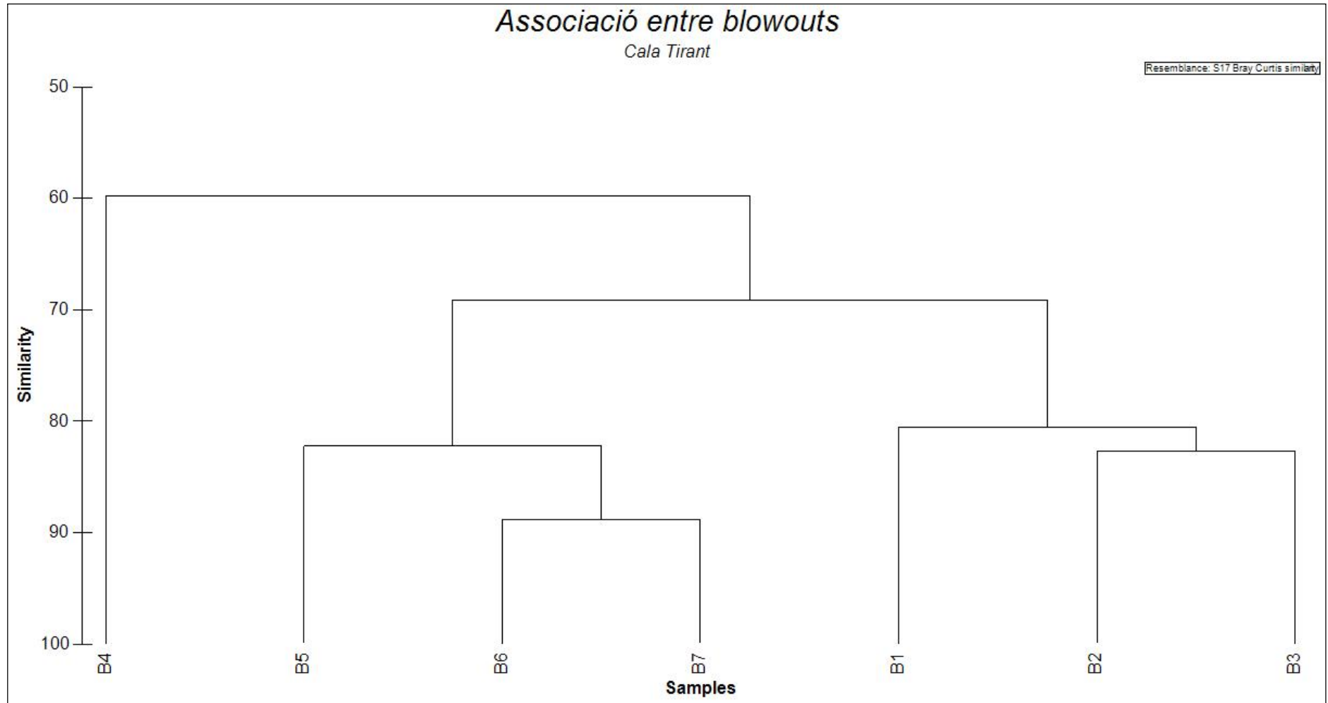
Figura 129: Anàlisi cluster dels 7 blowouts analitzats a Cala Tirant a partir de la consideració de les seves característiques geomorfològiques, ecològiques i estat de gestió..
