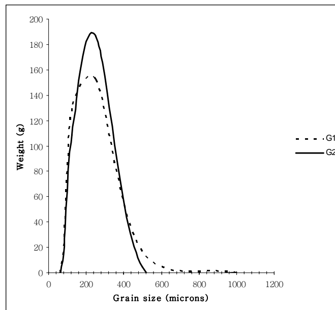
Figura 157: Distribució de la mida de gra en cada un dels punts mostrejats a partir de Folk i Ward (1957).
