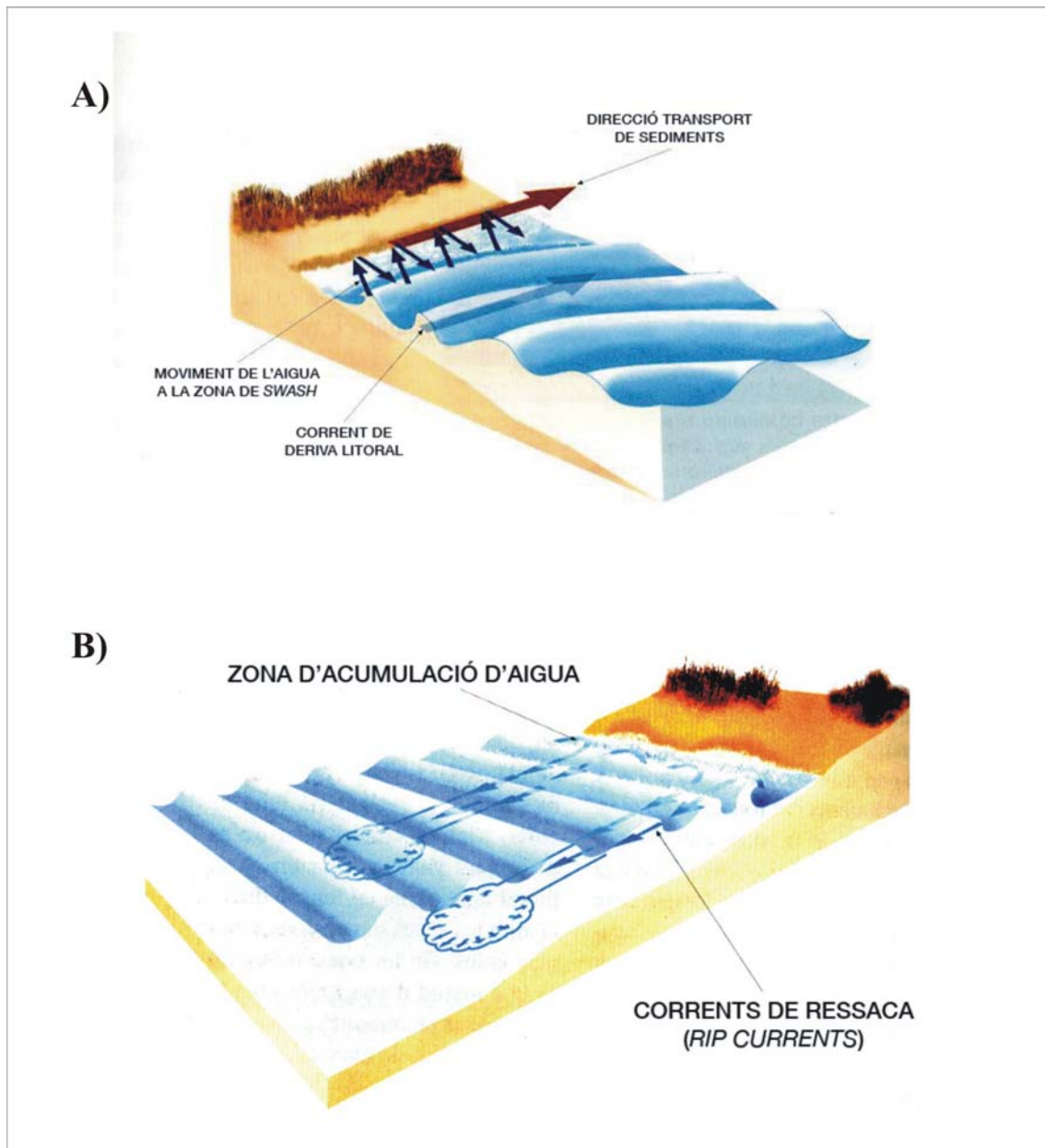
Figura 4: Els corrents marines són un dels agents mecànics més importants en tant a la configuració de les costes sedimentaries. Es poden distingir entre a) les corrents de deriva litoral, manco energètiques i paral·leles a la línia de costa, i b) les corrents de ressaca o rip currents , de retorn mar endins (Servera, 2004).
