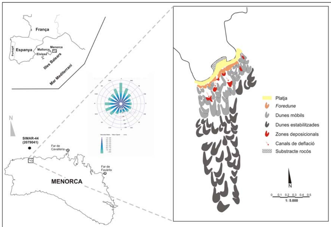
Figura 130: Localització geogràfica del sistema platja-duna de La Vall, i representació de les característiques geomorfològiques del sistema dunar.
