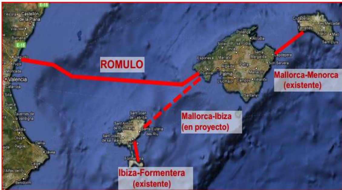
Esquema 5. Sistema de cableado eléctrico del Proyecto Rómulo, (2012). Fuente: Proyecto Rómulo. http://electronica.uc3m.es/geste/ROMULO.pdf
