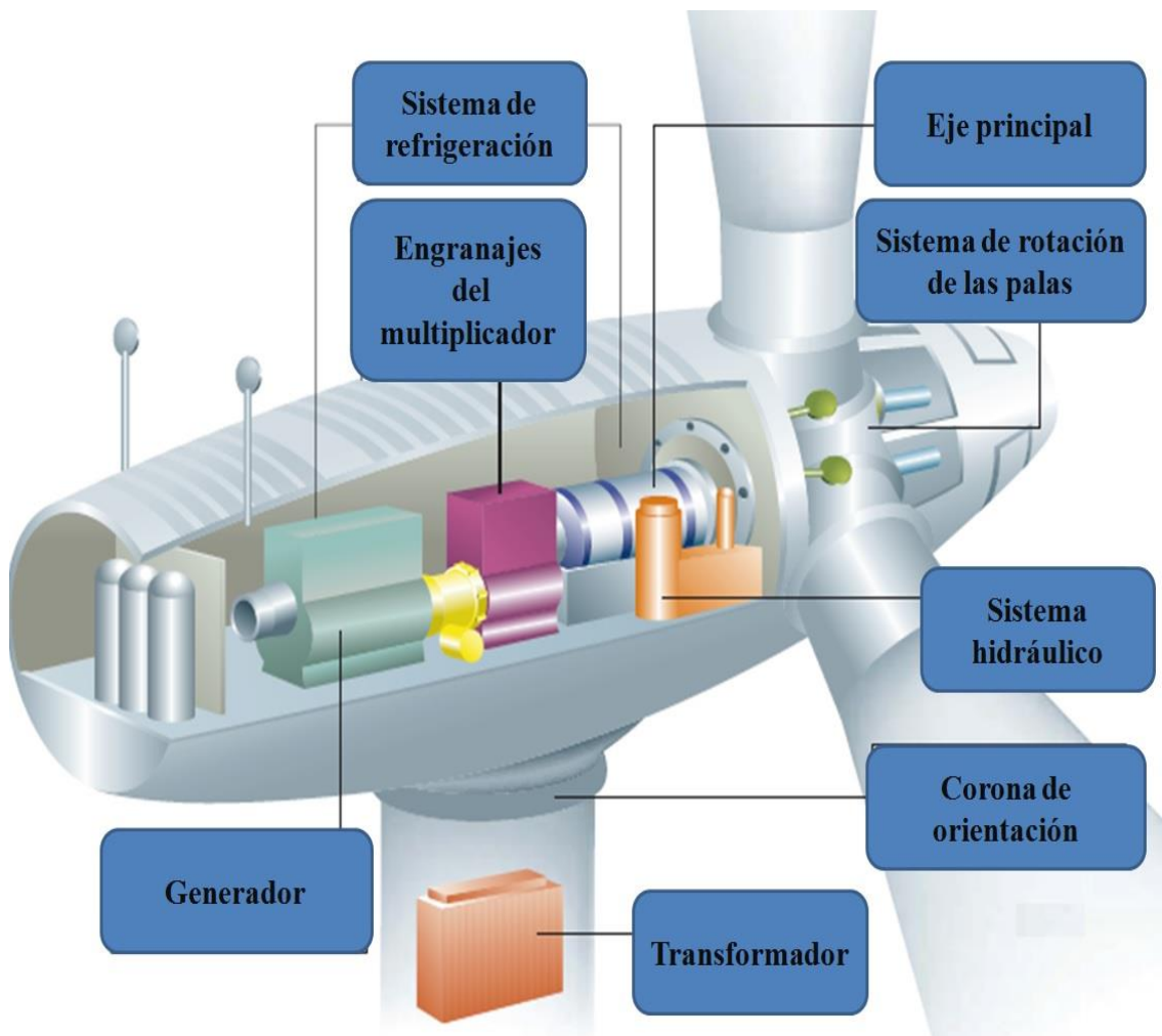
Esquema 10. Partes principales de un aerogenerador.
