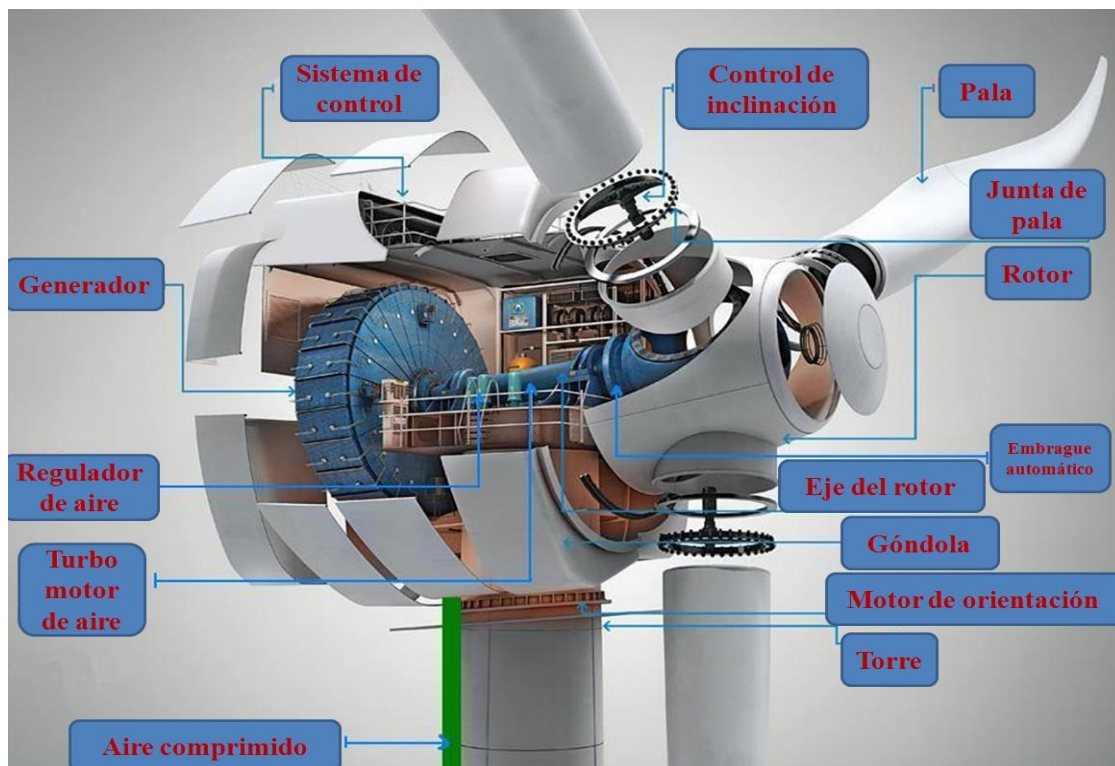
Esquema 9: Partes mecánicas de una turbina eólica.
