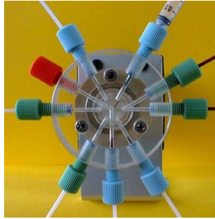
Figura 6. Fotografía del cabezal de un sistema LOV.
